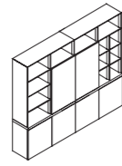
ED96 W2530•D430•H2130(mm)
