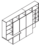
ED97 W3200•D560•H2130(mm)
