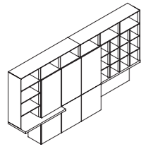
ED98 W3830•D560•H2130(mm)
